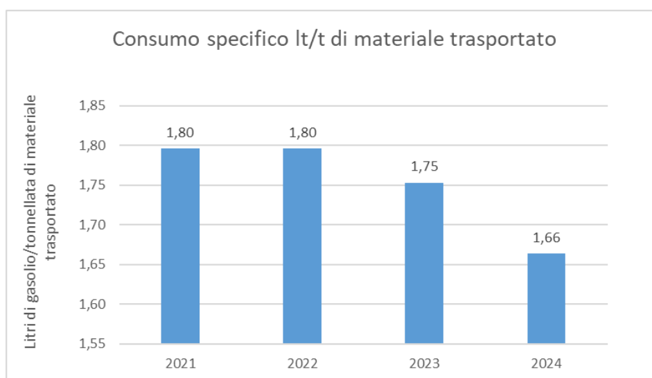
Fig. 14 – Andamento indicatore di prestazione ambientale "produzione" di Bernardelli Trasporti Srl.
